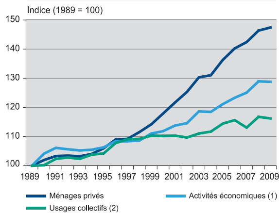
Consommation totale d'électricité, depuis 1989
