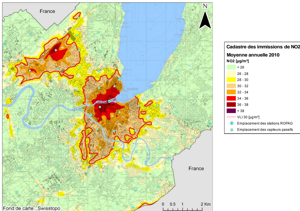
Figure 20. Carte des immissions de NO 2 sur l'agglomération genevoise pour 2010
