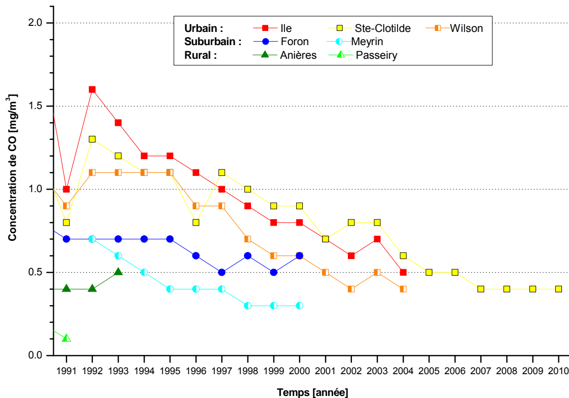
Figure 15. Concentration moyenne annuelle 8 de CO
