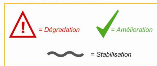
Figure 1. Bilan de la pollution de l'air par zone et par polluant, pour l'année 2010 ainsi que pour l'évolution sur la période 2003-2010
