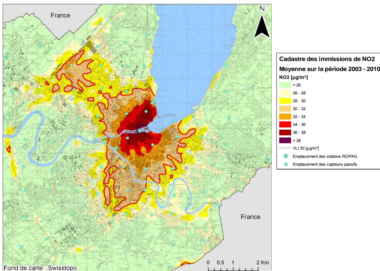
Figure 21. Carte des immissions moyennes de NO 2 sur l'agglomération genevoise pour la période 2003 à 2010
