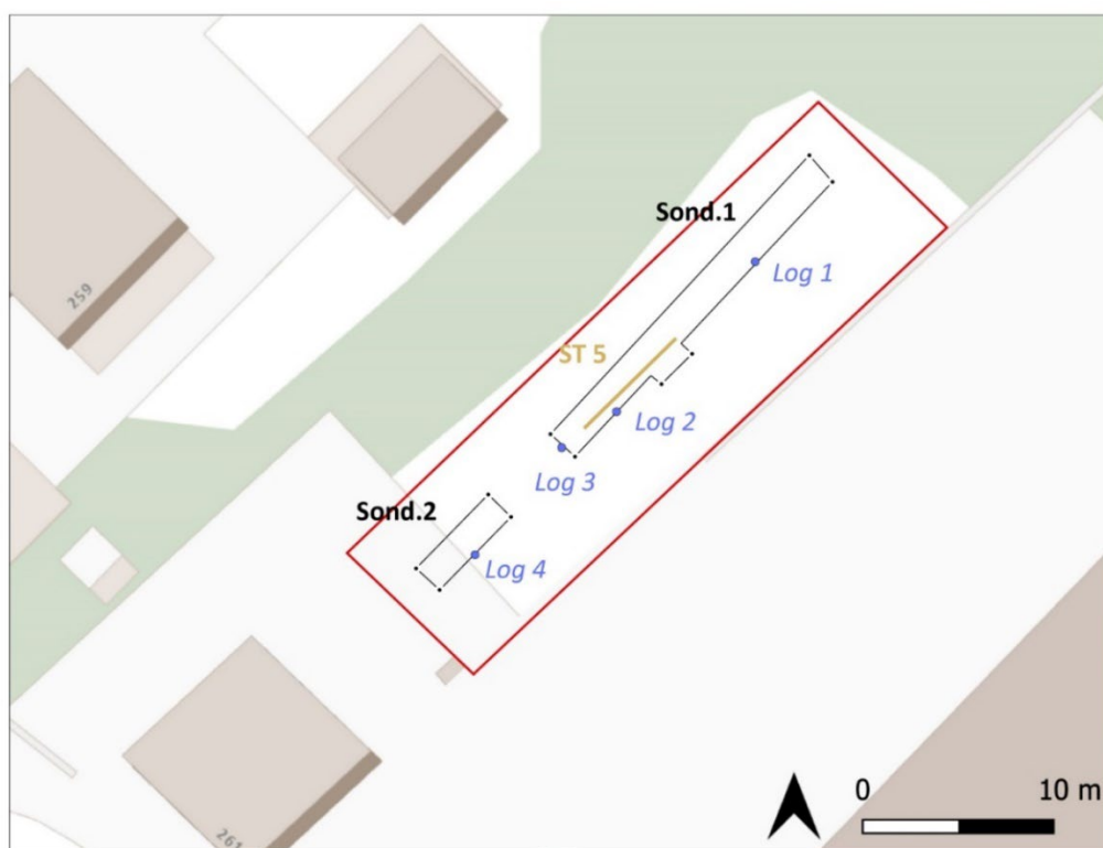
Fig. 4. Route de Veyrier 261 : implantation des sondages, des logs et des vestiges relevés.
