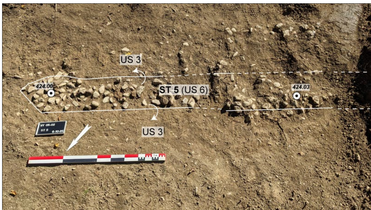
Fig. 9. Sondage 1 : vue en plan de la partie orientale du drain ST 5, à son niveau d'apparition.
