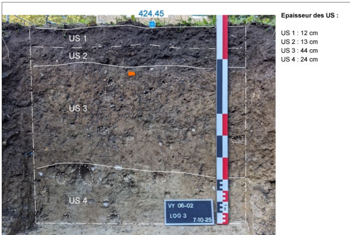
Fig. 7. Sondage 1, log 3 : relevé des unités stratigraphiques. Vue en direction du sud-ouest. En orange : fragment de terre cuite.
