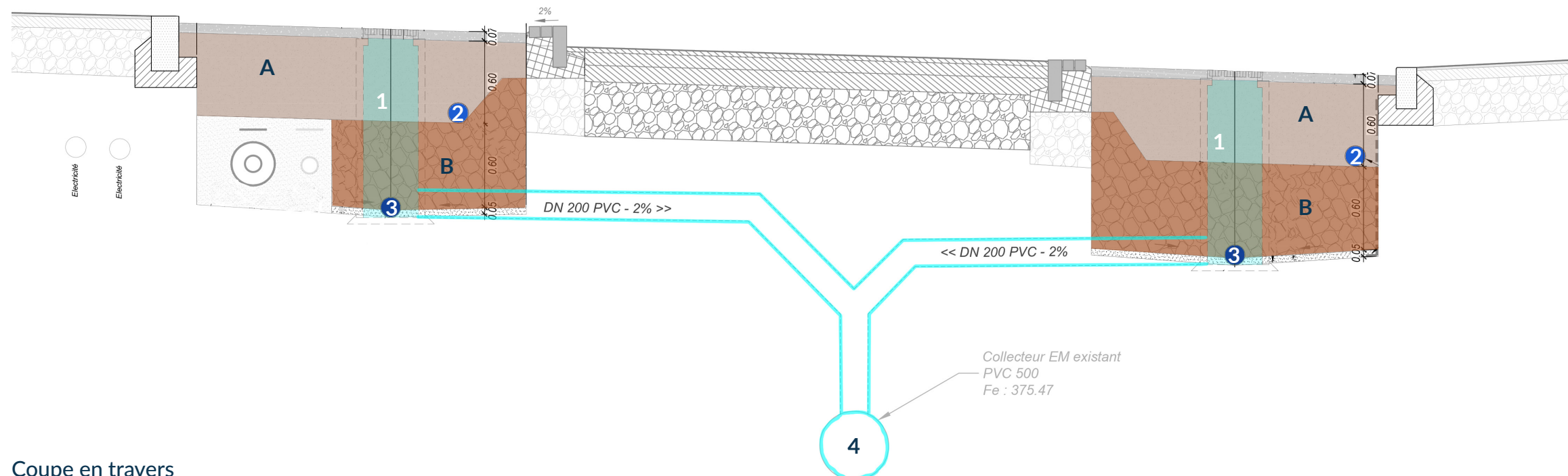
Drain d'aération et de diffusion (-60cm)
