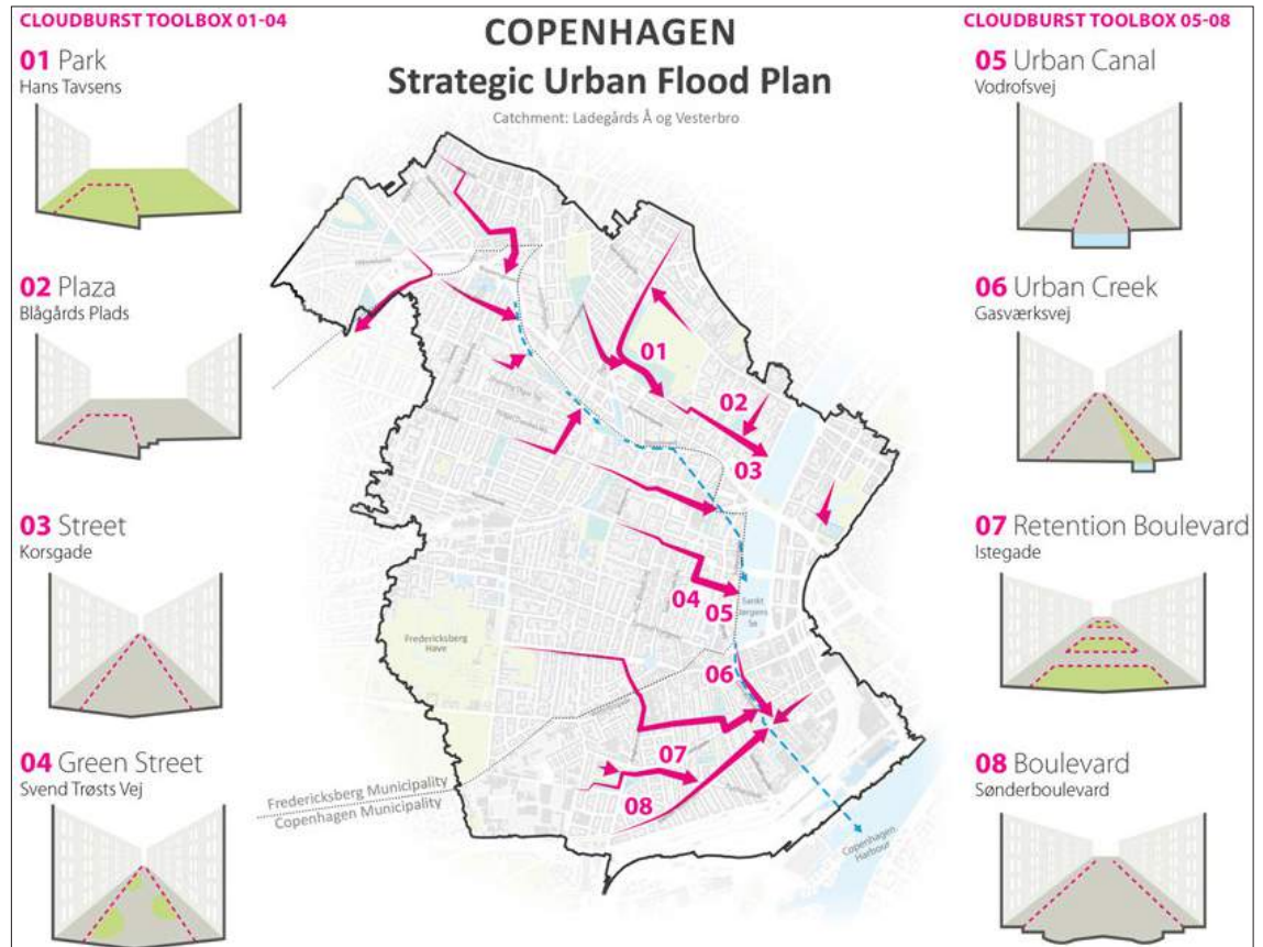
Fig. 22 Schéma d'évacuation des événements extrêmes et toolbox des types d'intervention suivant la morphologie urbaine existante. ©Ramboll Studio Dreiseitl
