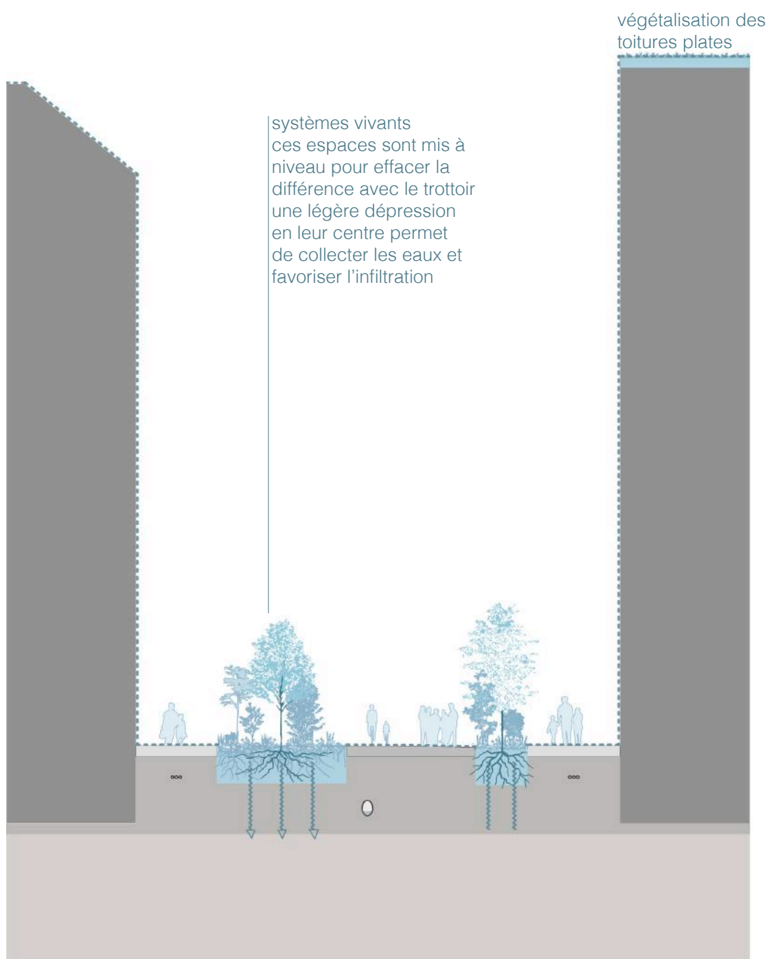
Fig. 111 Coupe de principe Étape 2. coupe au 1/200 ème
