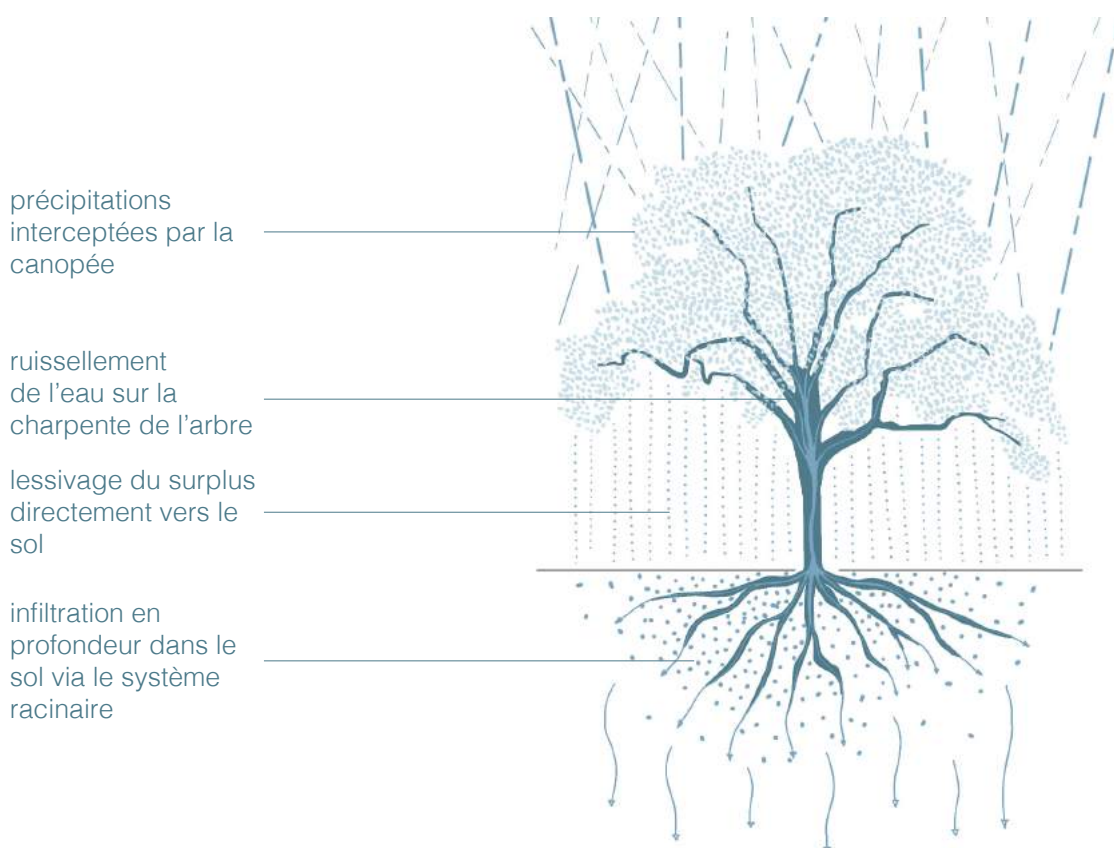
Fig. 5 L'interception de la pluie et la conduite dans le sol via la structure de l'arbre
