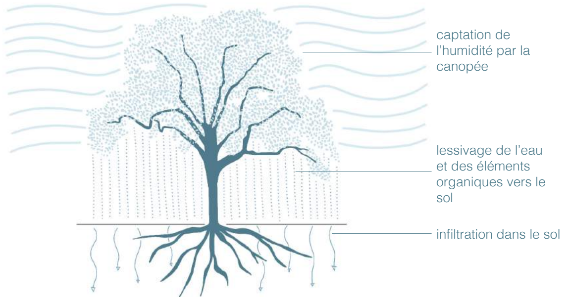
Fig. 6 La captation de l'humidité de l'air et la précipitation de l'eau au sol
